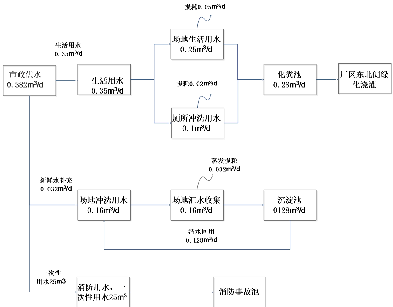
水平衡图
